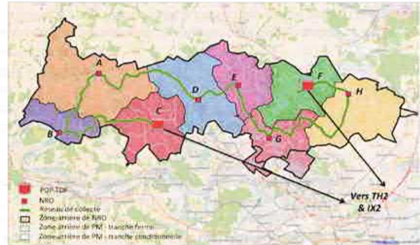
Réseau de collecte du RIP VORTEX
